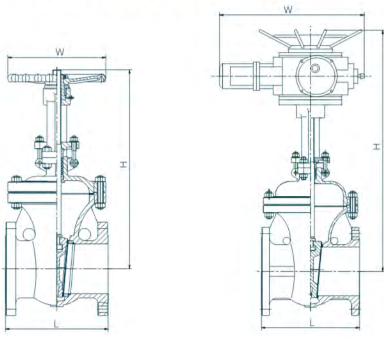
尺寸及重量Size & weight Class 300
