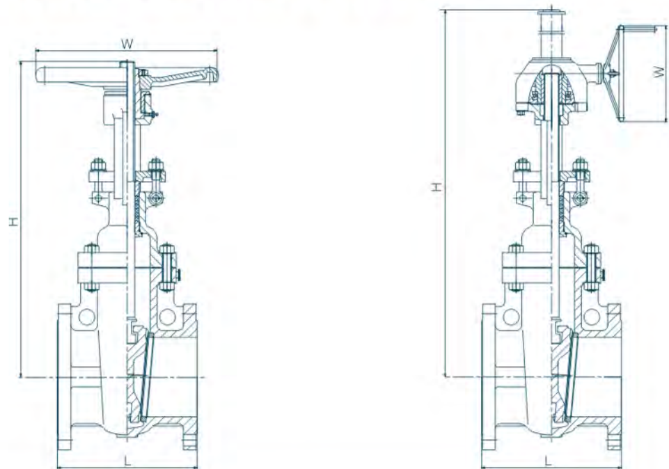
尺寸及重量Size & weight Class 150
