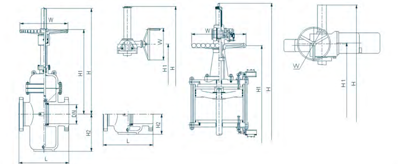
主要外形尺寸Main Size of outside PN6.4MPa
