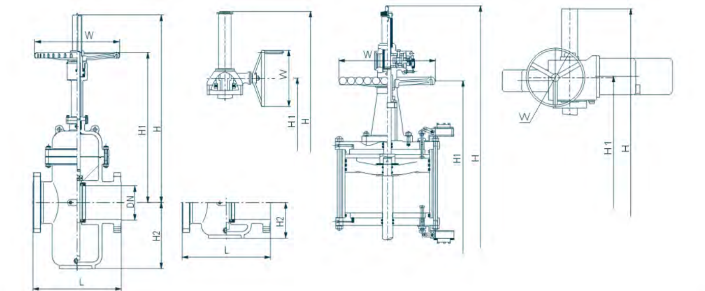
主要外形尺寸Main Size of outside Class400
